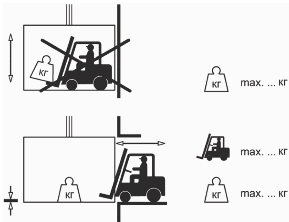
Рисунок 14 - Пиктограмма на посадочных площадках для погрузочно-разгрузочных устройств
