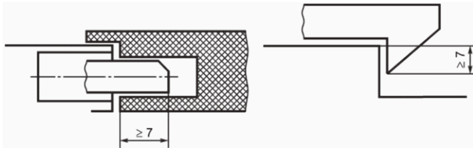
Рисунок 12 - Примеры запирающих элементов
