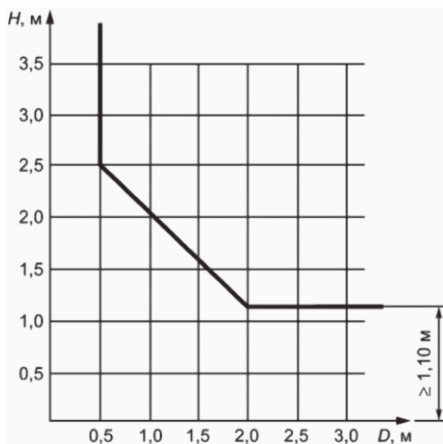
Рисунок 2 - Частично огражденная шахта - расстояние до движущихся частей лифта
