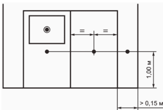
ж - полностью собранная дверь шахты со створками двери и боковыми рамами (пример соответствует рисункам 11 а и 11 б)
