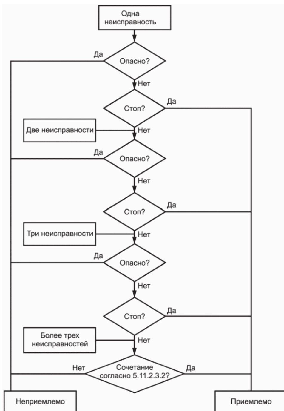
Рисунок 25 - Блок-схема оценки цепи безопасности
