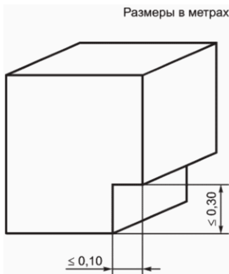
Рисунок 4 - Максимальные уменьшения пространств безопасности для персонала
