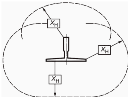
Рисунок 6 - Горизонтальное расстояние X_H вокруг направляющей
