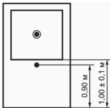
д - створка двери со стеклянной панелью на высоте более 1,0 м
